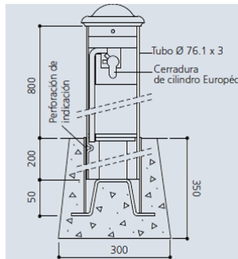
ESQUEMA DE INSTALACIÓN
